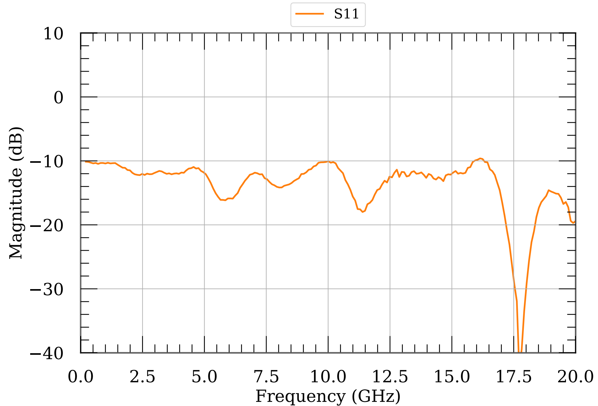
LNA S-params module033v2
